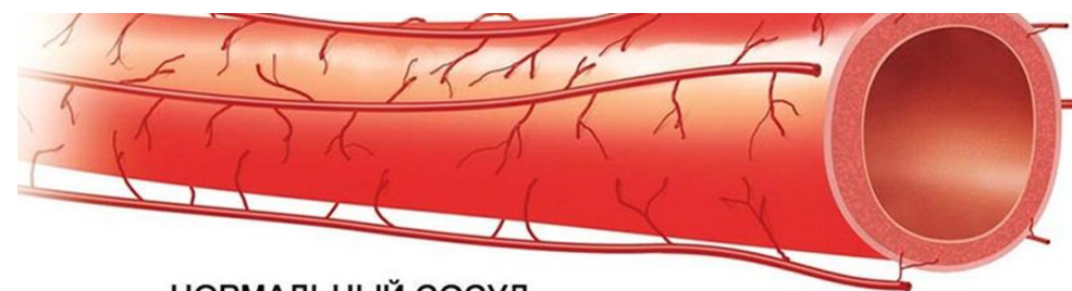
НОРМАЛЬНЫЙ СОСУД
