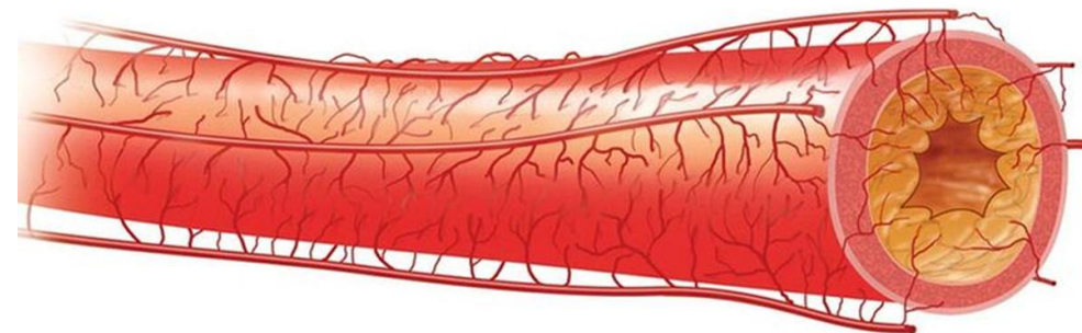
АТЕРОСКЛЕРОЗ
